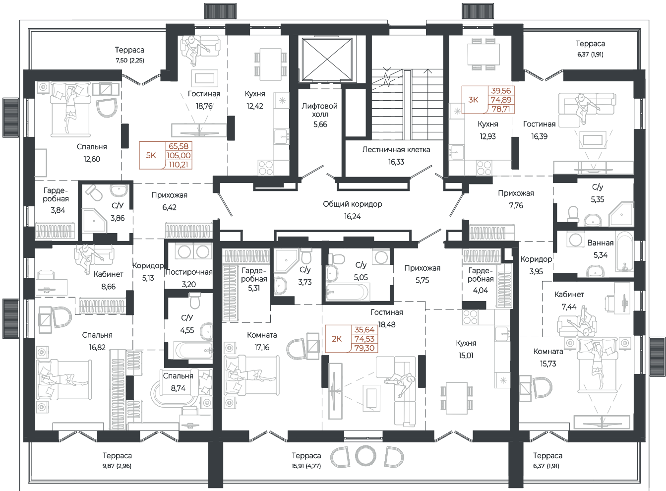
6 ЭТАЖ
