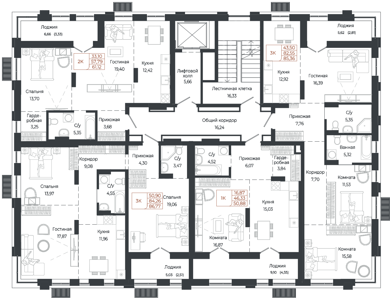
5 ЭТАЖ
